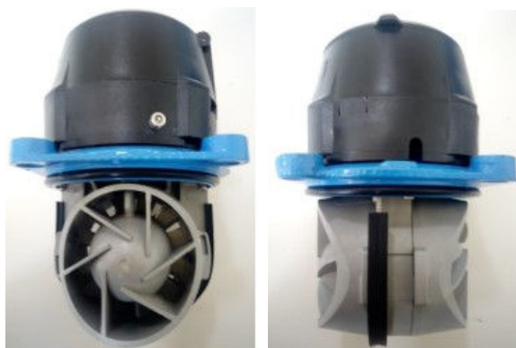
Foto 4. Mecanismo del contador
